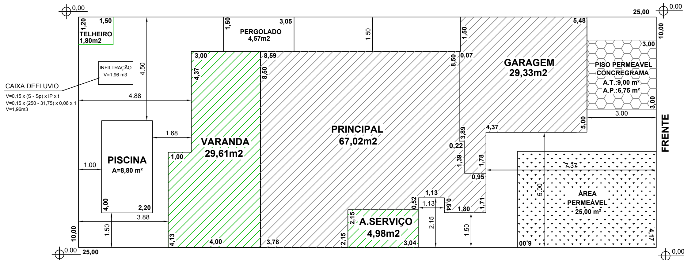
PLANTA PAV. TÉRREO escala 1:100
