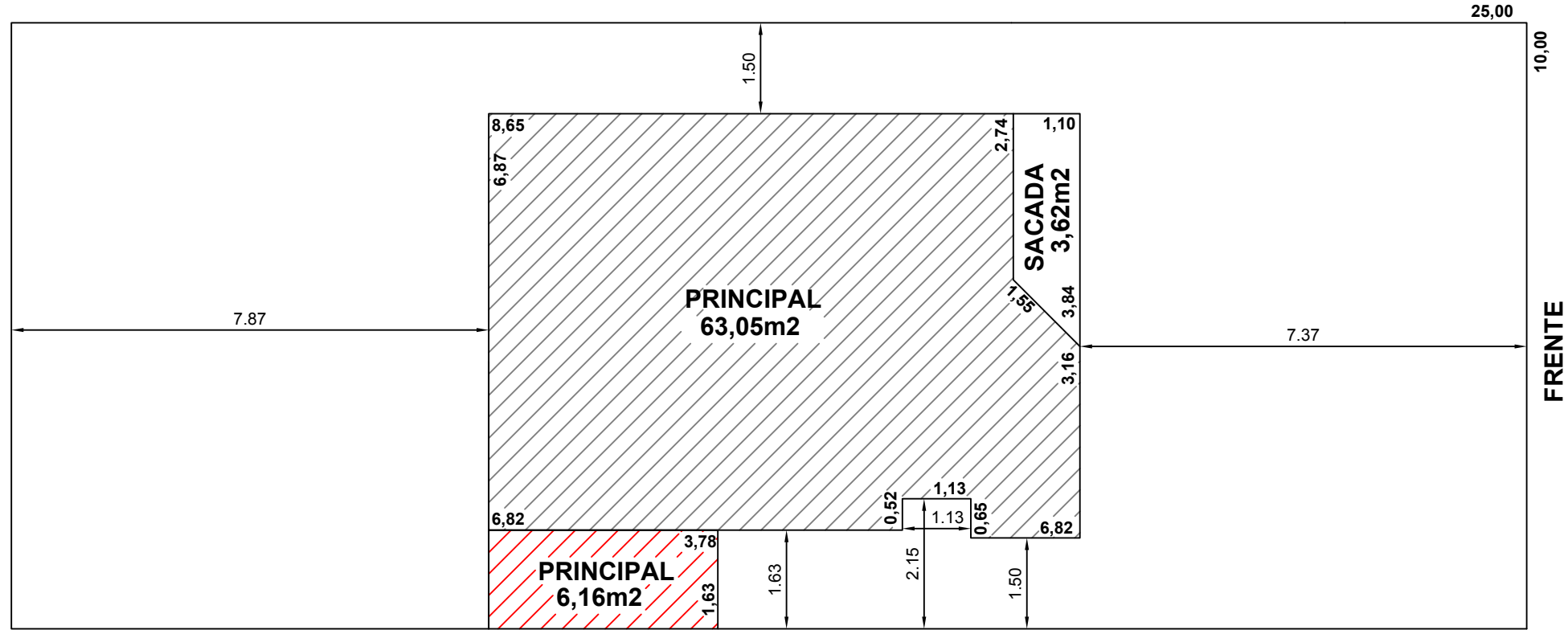
PLANTA PAV. SUPERIOR escala 1:100
