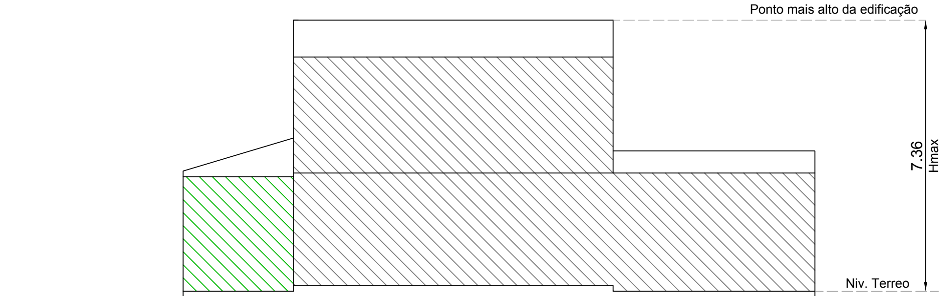
CORTE ESQUEMATICO escala 1:100
